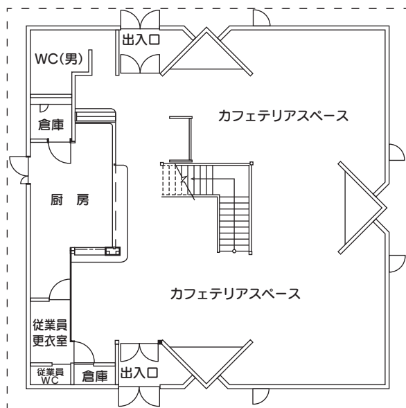
1階 平面図
